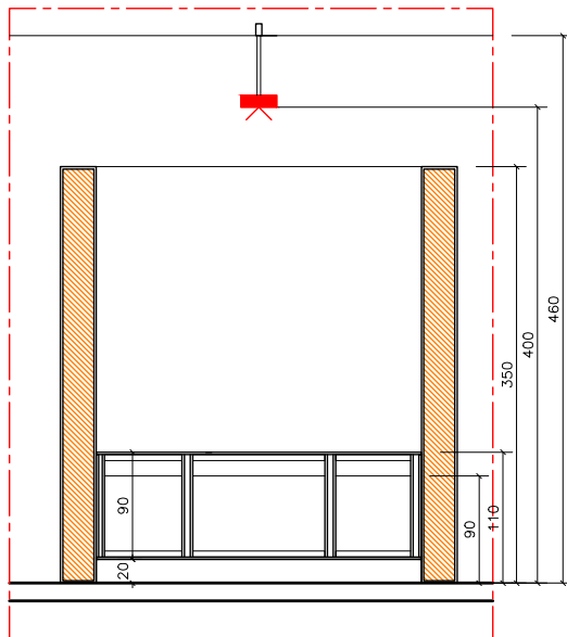
COUPE AA ECH 1:50
