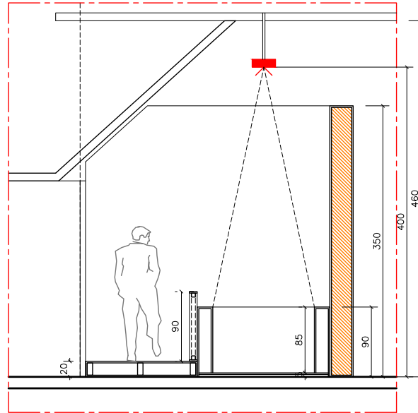
COUPE BB ECH 1:50
