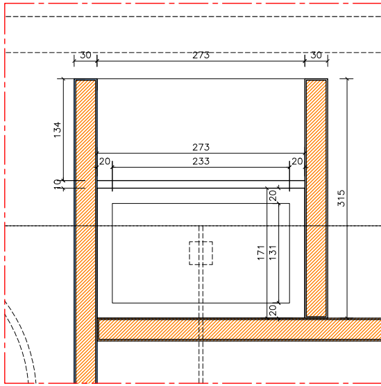
PLAN ECH 1:50
