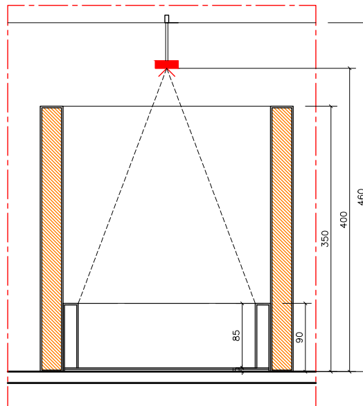
COUPE CC ECH 1:50
